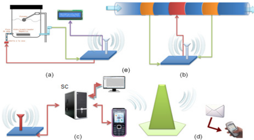
Figura 3. Arquitectura de AIDA
