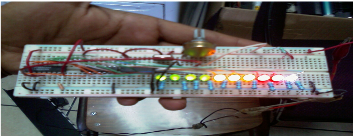
Figura 8. Circuito medidor de agua
