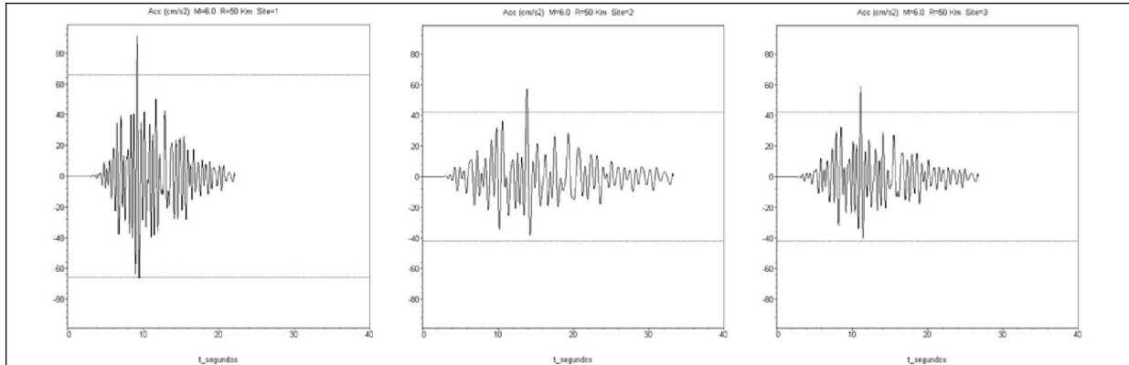
Figura 4. Componente horizontal de los acelerogramas sintéticos calculado para una magnitud 6.0 a una distancia epicentral de 50 km, de izquierda a derecha: sobre sedimentos superficiales (espesor menor de 20 metros), sobre sedimentos profundos (espesor mayor de 20 metros), y sobre roca
