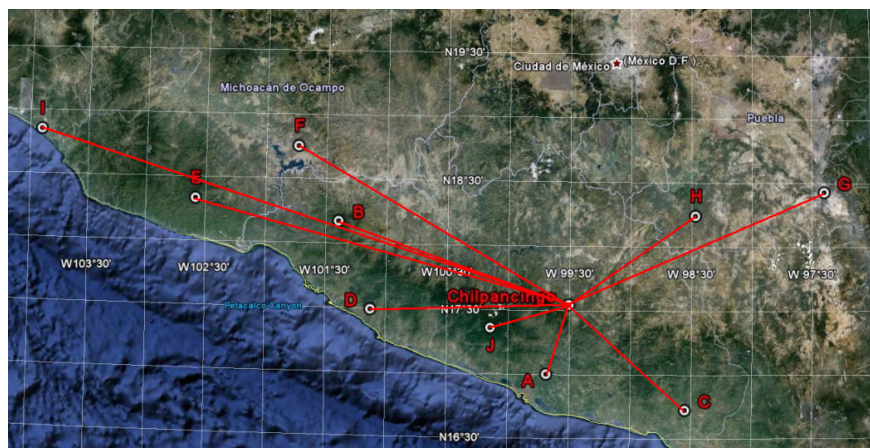
Figura 4. Mapa de localización de los epicentros de los sismos más intensos
